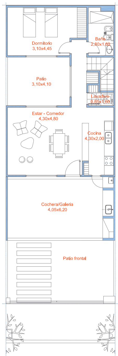
Planta baja
