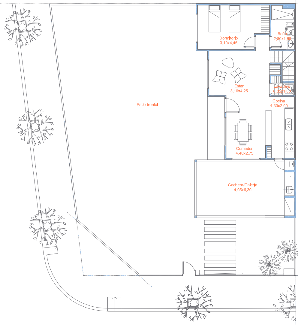
Planta baja
